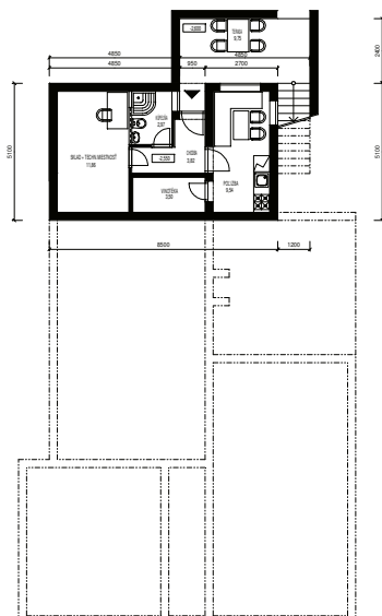
PODORYS SUTERÉNU
