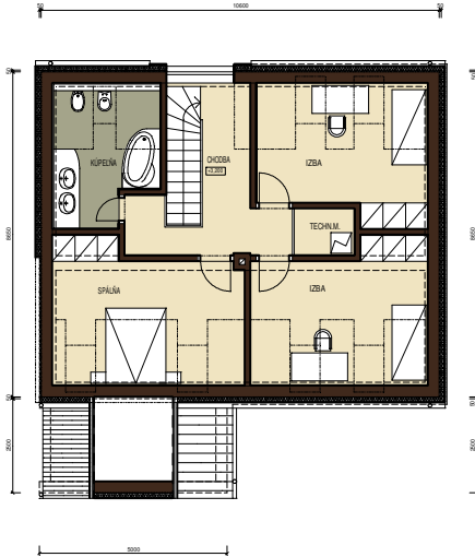
PODORYS PODKROVIA
