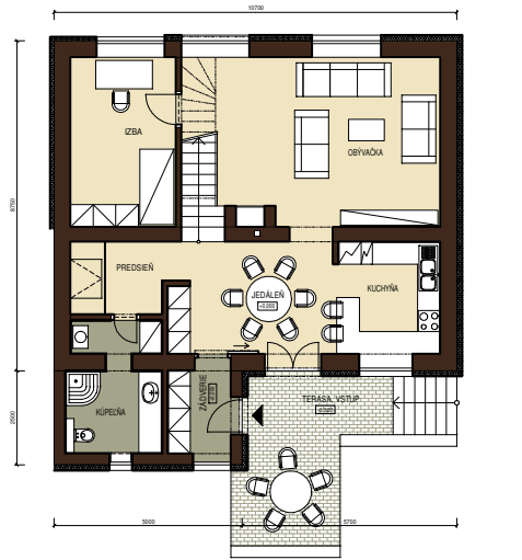
PODORYS PRÍZEMIA
