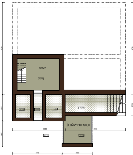
PODORYS SUTERÉNU
