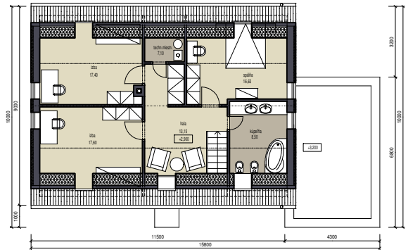
PODORYS PODKROVIA
