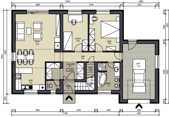
PODORYS PRÍZEMIA
